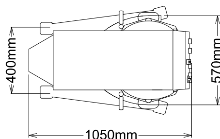
Boven aanzicht
